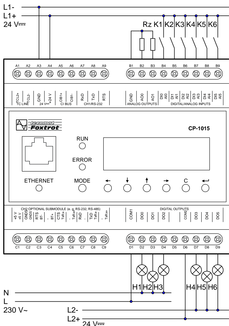
Obr. 4.1 Základní zapojení modulu CP-1015
