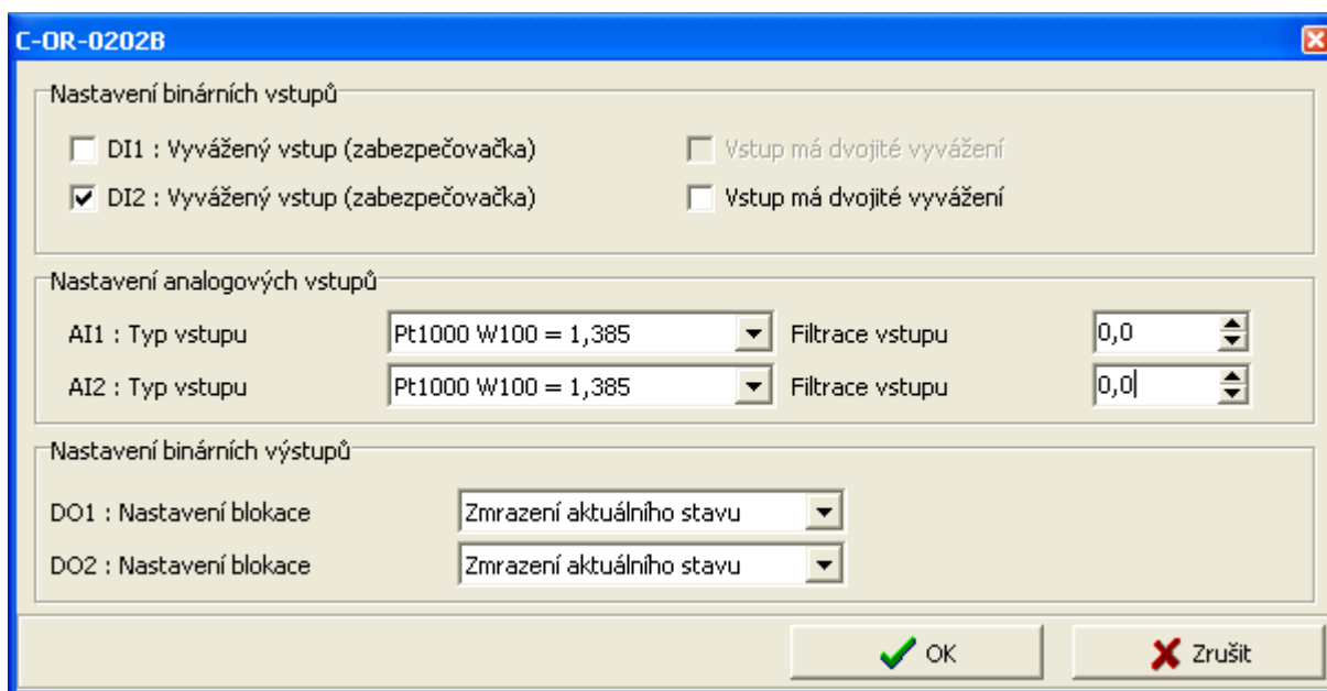
Fig. 3.65 Module configuration
