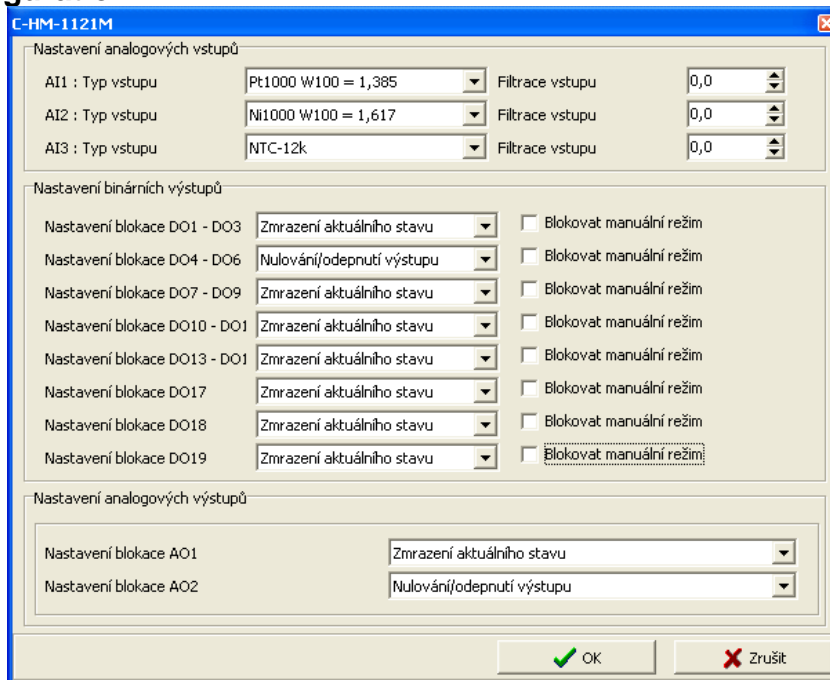
Fig. 3.11 Module configuration
