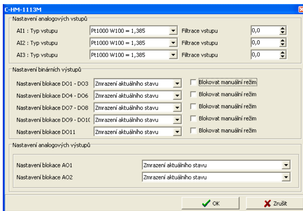
Fig. 3.8 Module configuration
