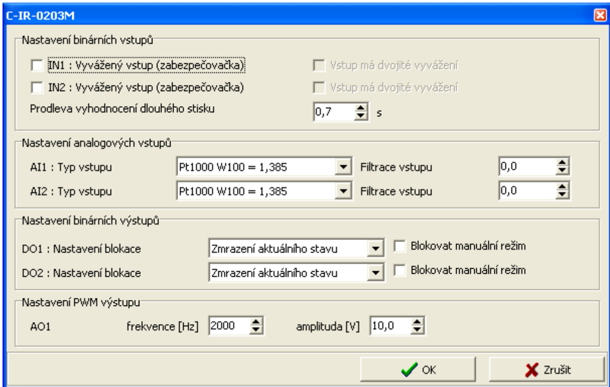
Fig. 3.27 Module configuration
