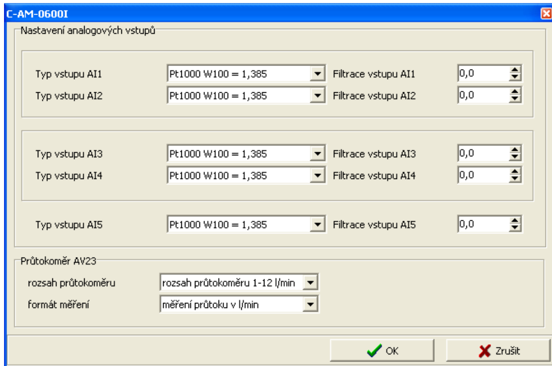
Fig. 3.2 Module configuration
