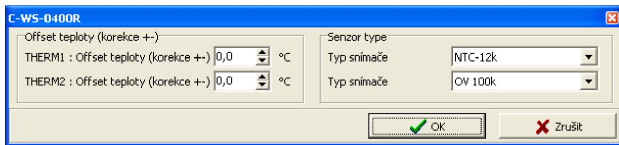
Fig. 3.86 Module configuration
