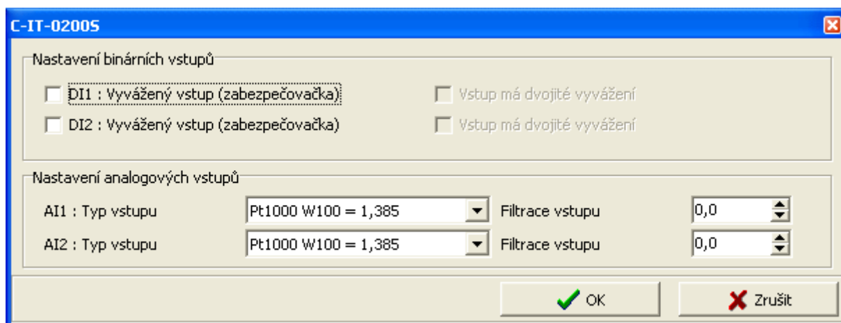
Fig. 3.46 Module configuration
