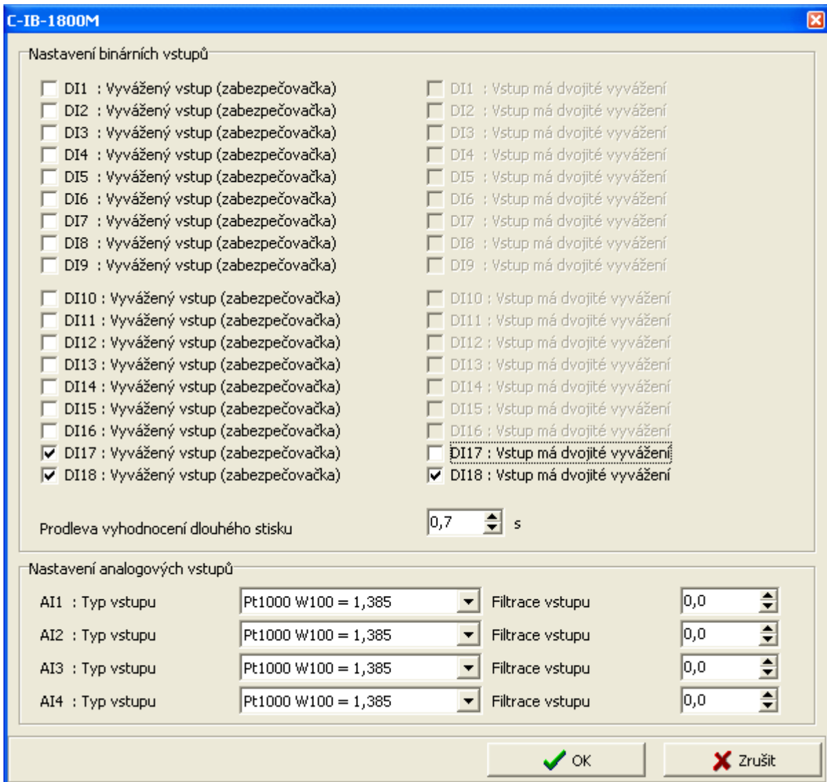
Fig. 3.16 Module configuration
