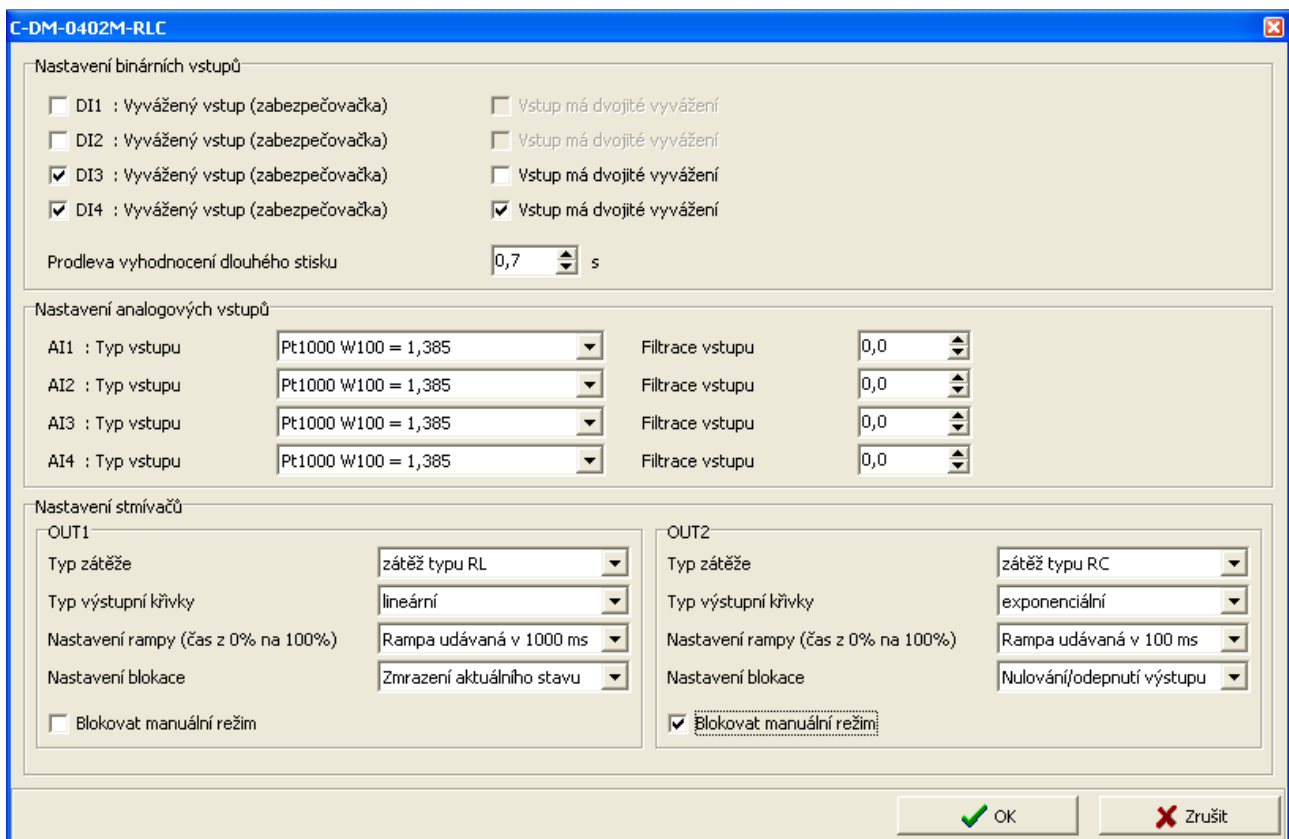
Fig. 3.28 Module configuration
